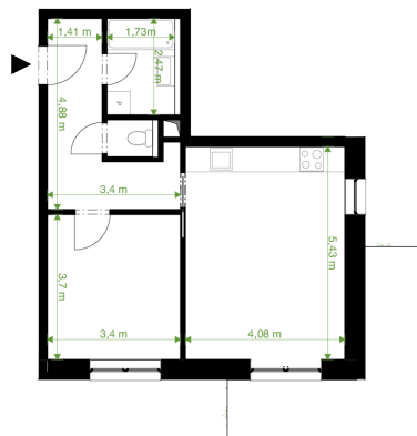
Orientační rozměry
