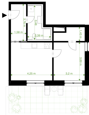
Orientační rozměry
