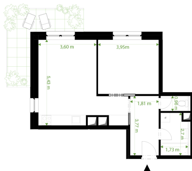
Orientační rozměry
